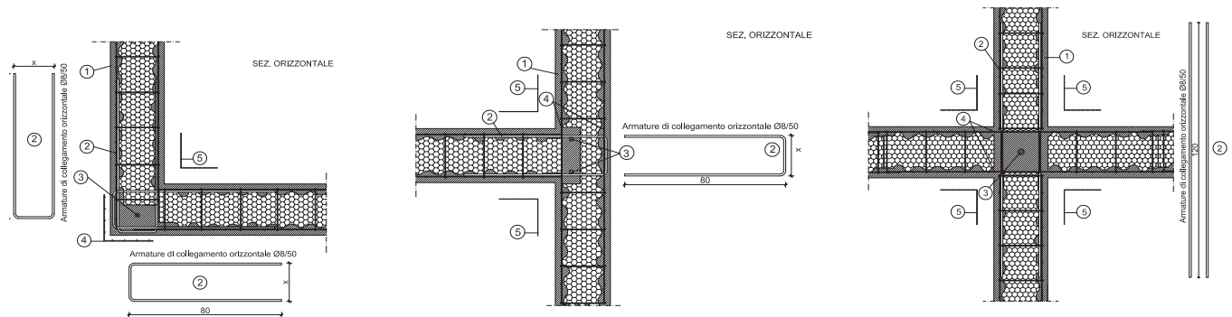
Nodo a 2 vie
