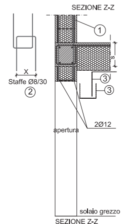
Incatenamento per porta
